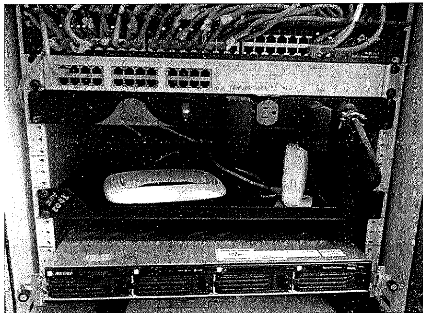
IMAGEN: Se puede visualizar router, modem, Switch y servidor buffalo.
